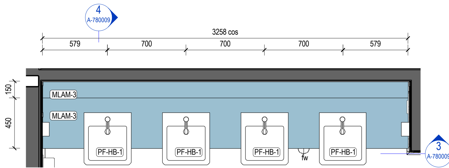
2 JO-BW-8 Plan 1 : 20
