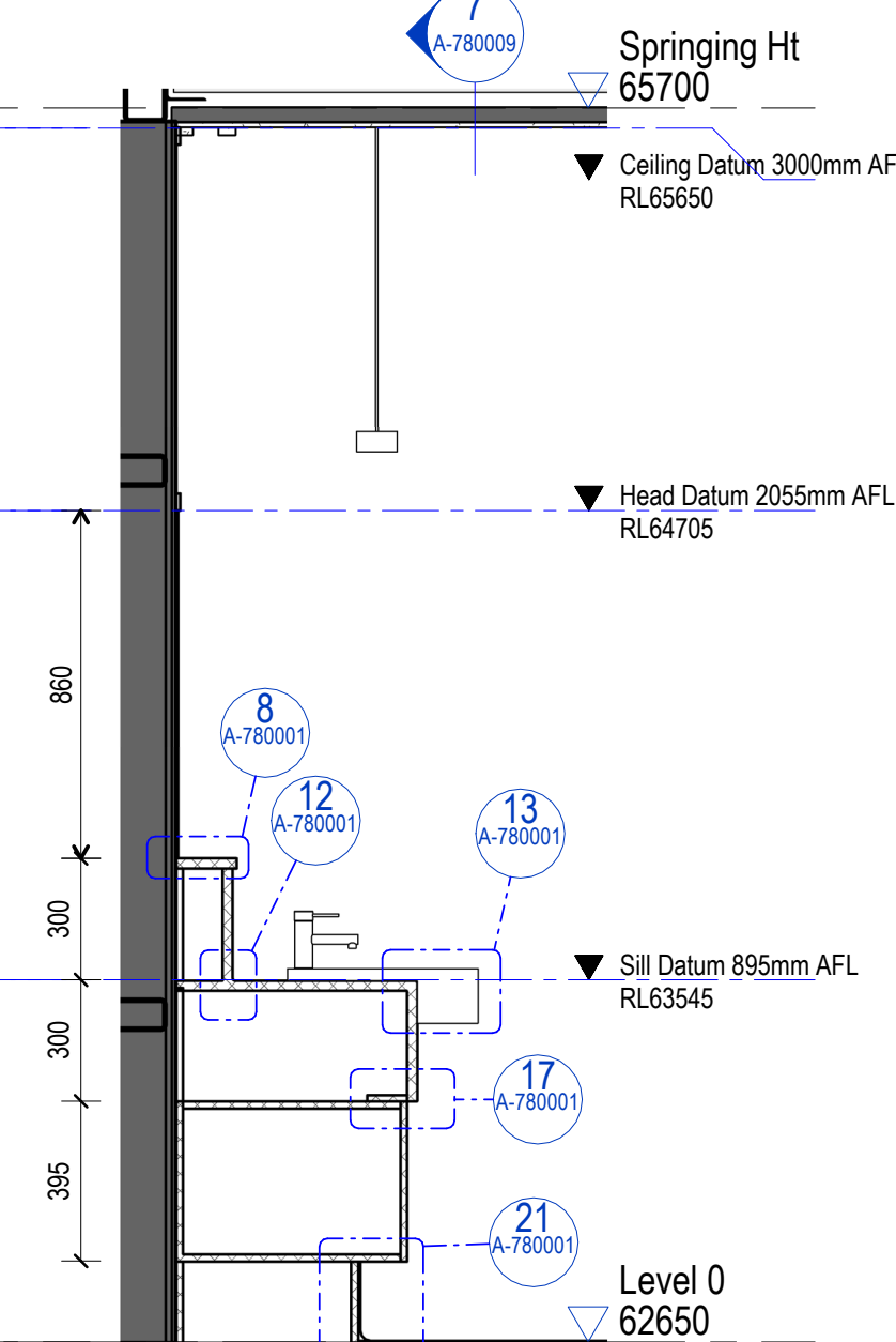
8 JO-BW-9 Section 1 : 20
