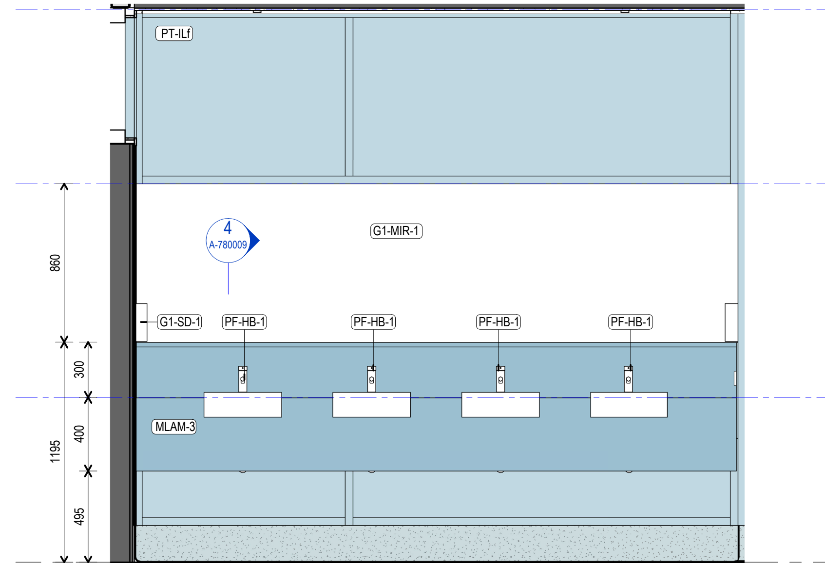
3 JO-BW-8 Elevation 1 : 20
