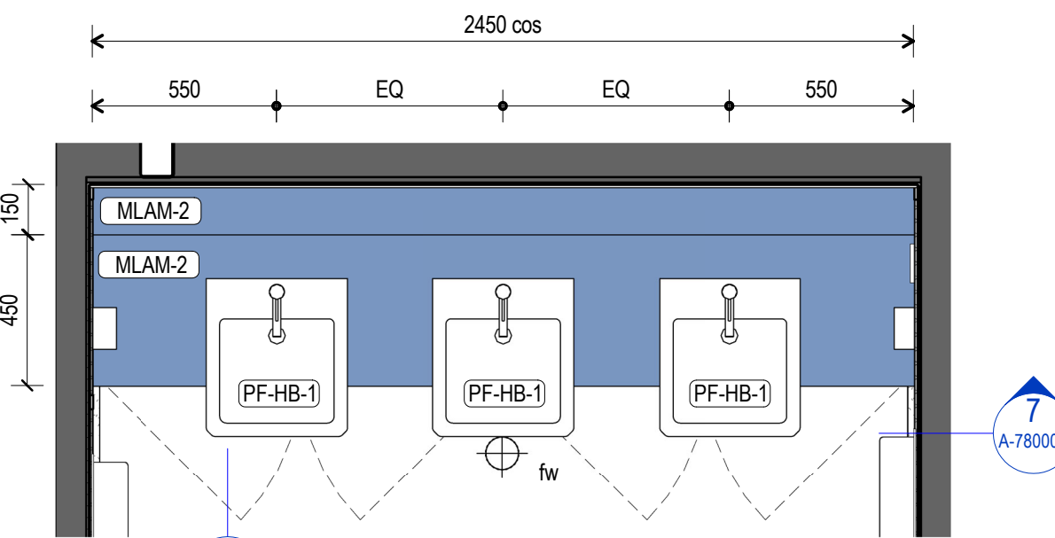
3 JO-BW-8 Elevation 1 : 20
