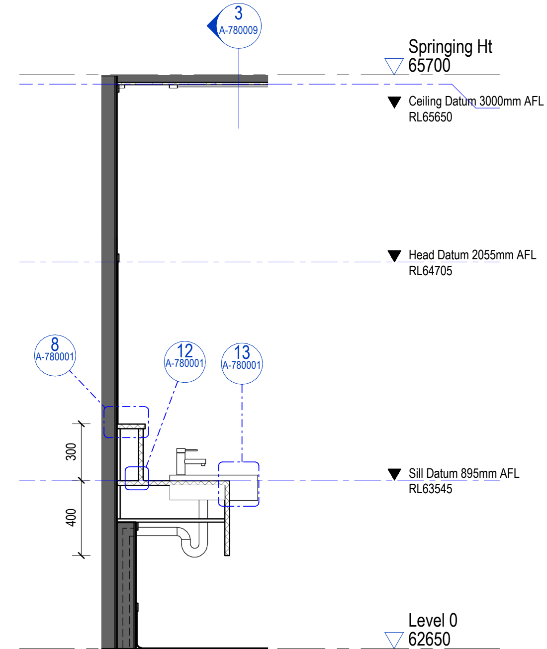
4 JO-BW-8 Section 1 : 20
